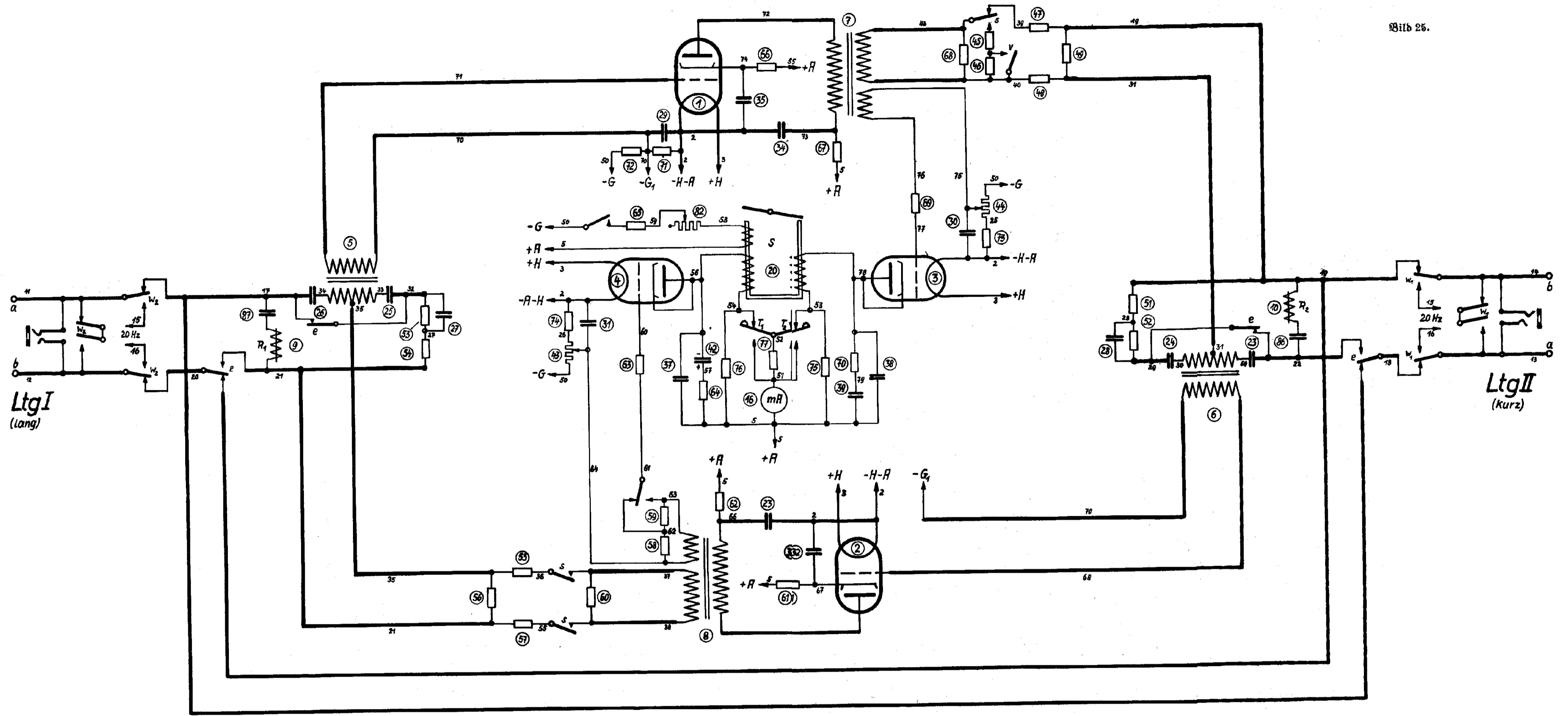
Gesamtschaltbild Feldverstärker a
