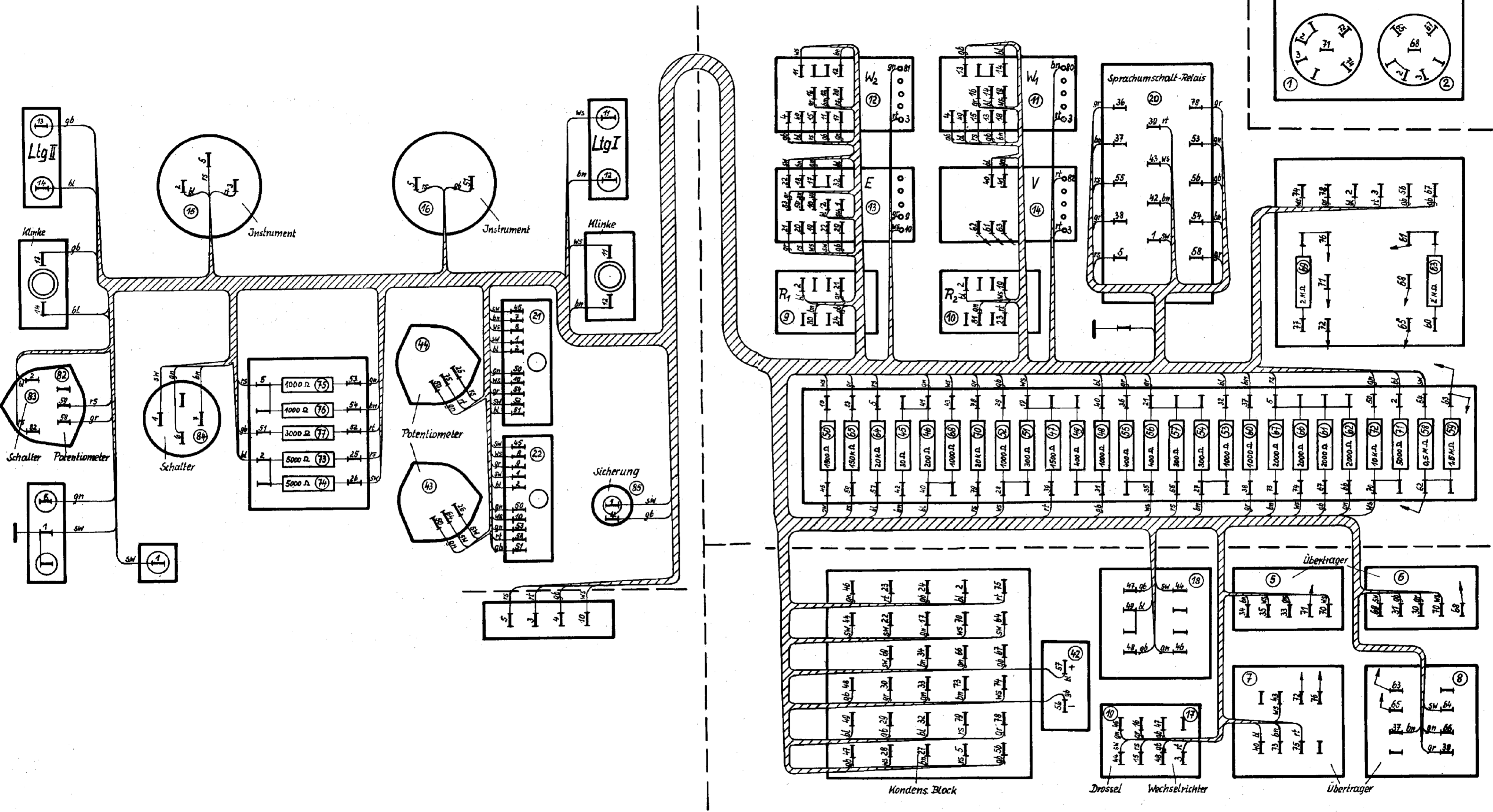
Verdrahtungsplan für den Feldverstärker a
