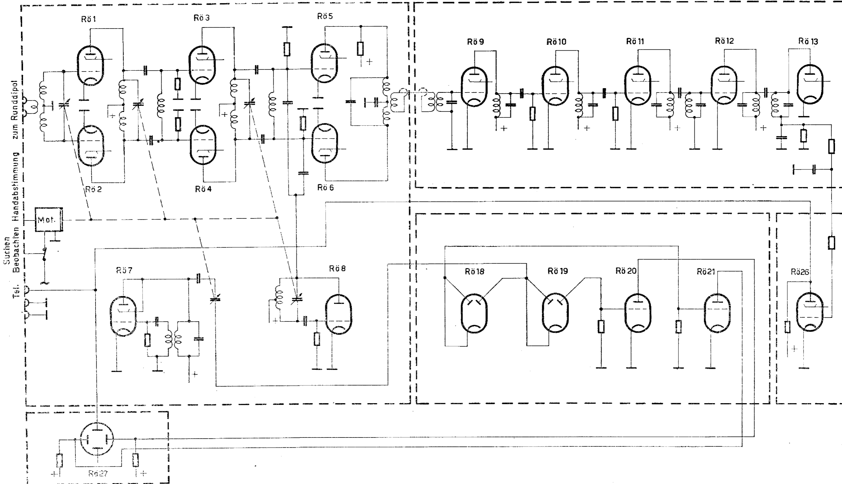
Prinzipschaltbild
