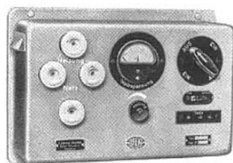
Bedienungsgerät für Dreiphasen-Anlagen
