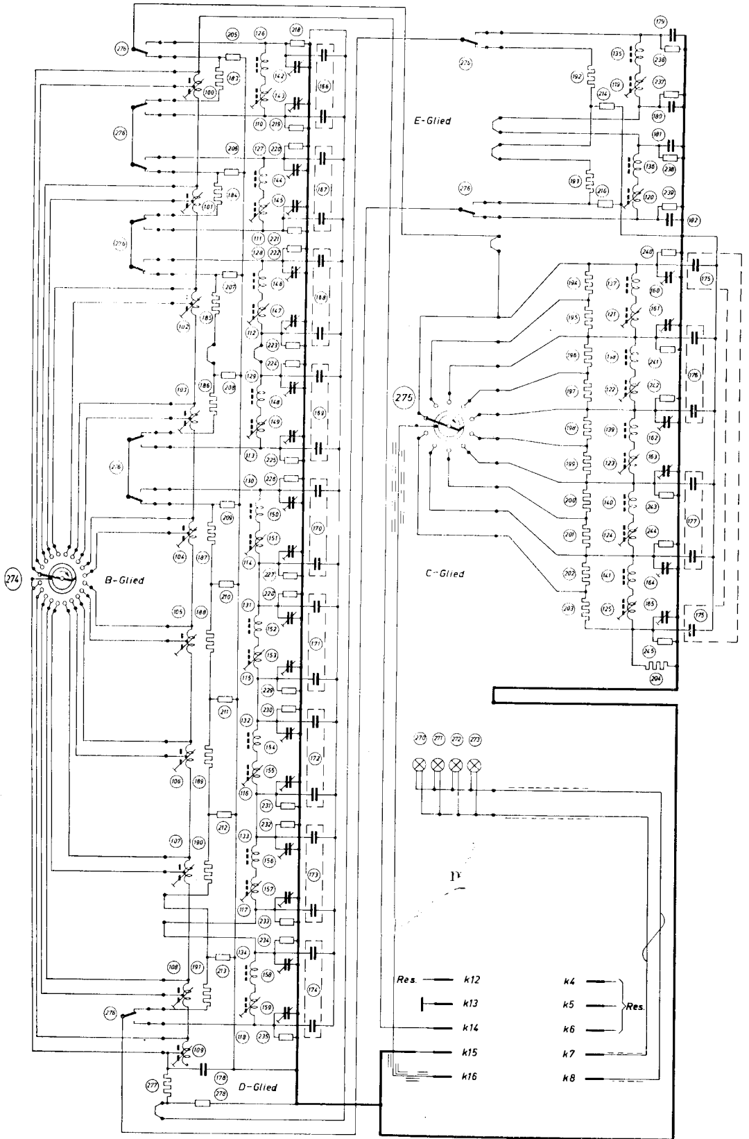
Schaltbild vom Einsatz OK
