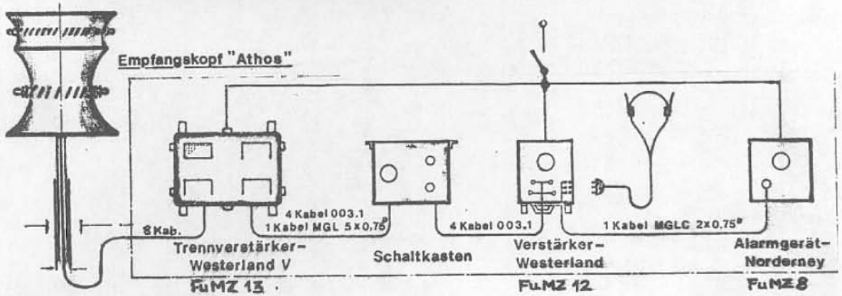
Sektorperilanlage FuMB 35 "Athos" (1,5 - 15 GHz)
