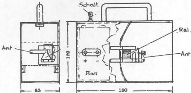
CMW-Prüfsender FuMZ 10 "Puck 901" für \lambda = 10 cm
