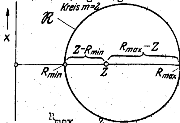
Ortskurve des Widerstandes im Leitungsdiagramm
